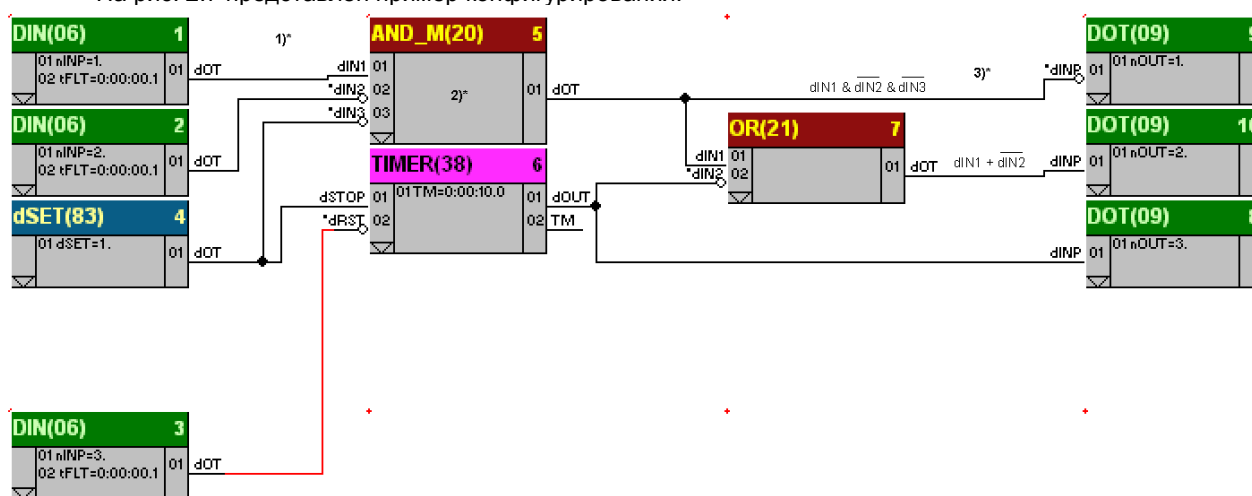
Рисунок 2.7 - Пример конфигурирования
