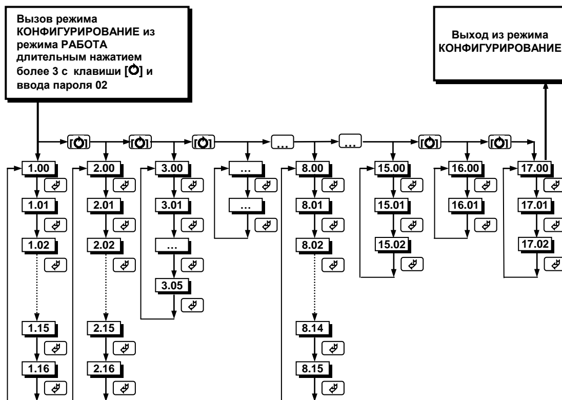
Рисунок 4.2 - Диаграмма уровней режима конфигурации и настроек
