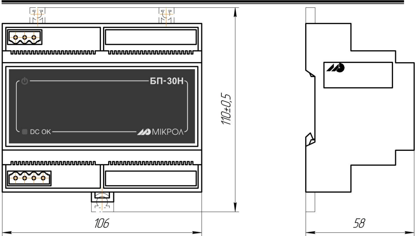
Рисунок 1.1 – Внешний вид и габаритные размеры БП-30Н-1к
