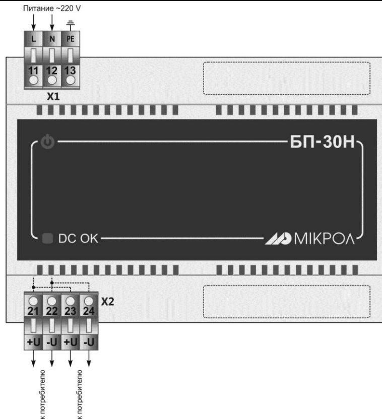
Рисунок 3.2 – Схема внешних соединений БП-30Н-1к
