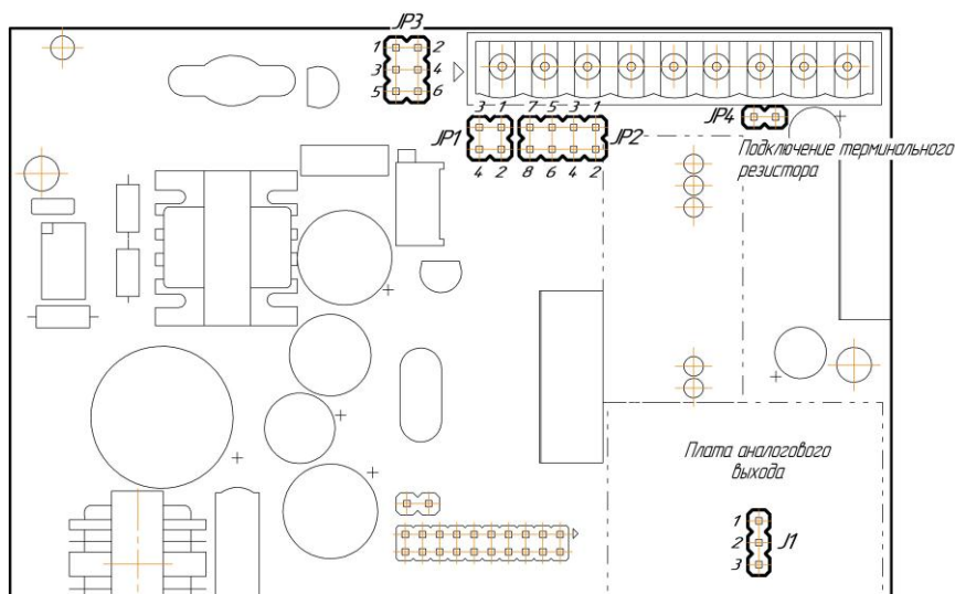
Рисунок 4.2 – Положение перемычек на плате процессора и на модуле аналогового выхода
