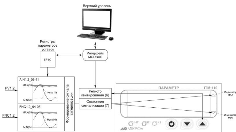
Рисунок 3.6 – Блок-схема блока сигнализации
